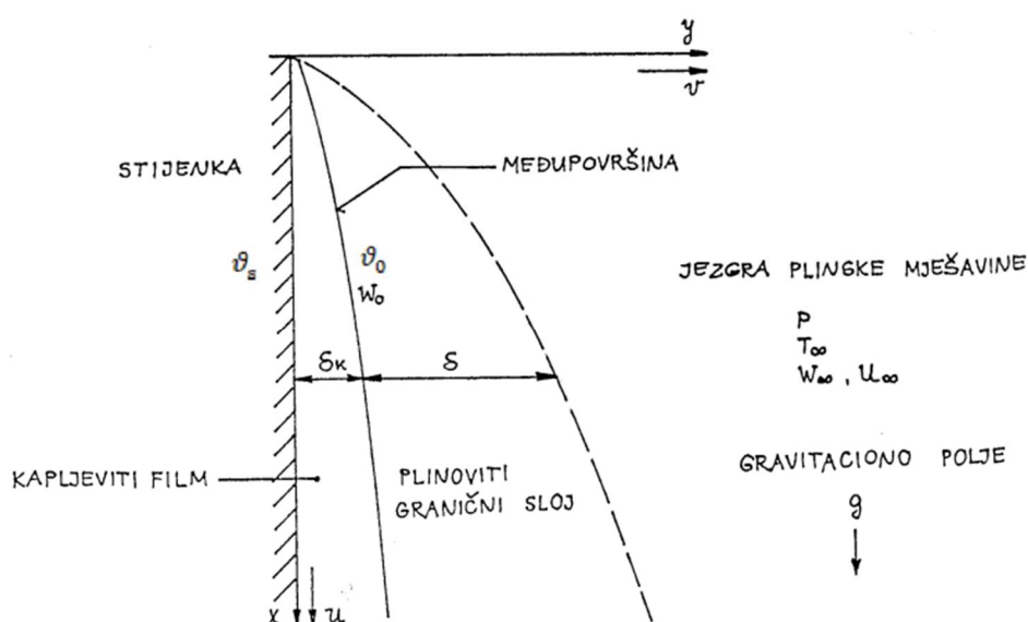
Slika 7. Fizikalni model kondenzacije vodene pare i zraka [50]
