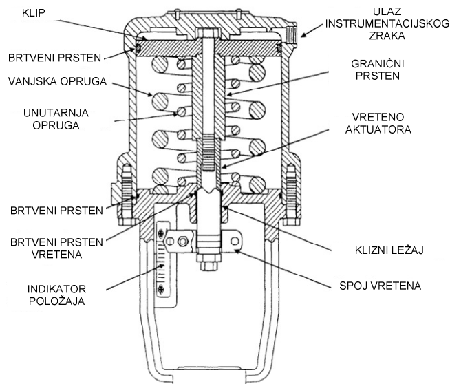
Slika 6.3 Cilindar aktuator s oprugom
