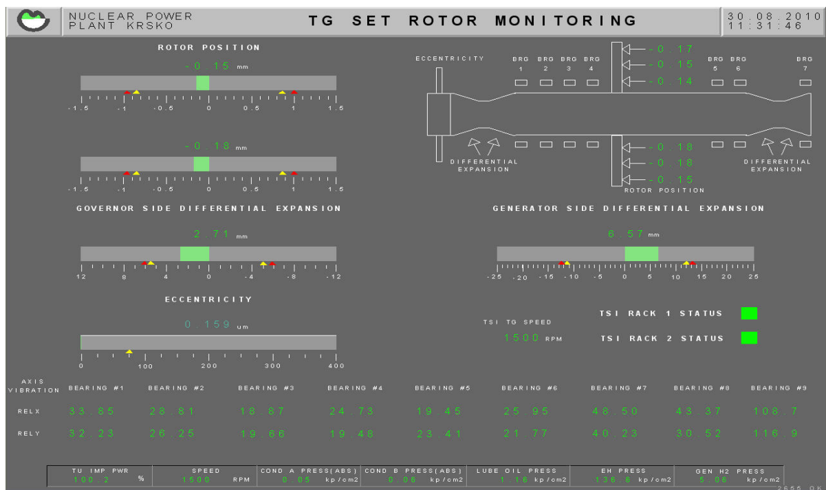
Slika 4.5 Kontinuirani monitoring generatora NEK-a
