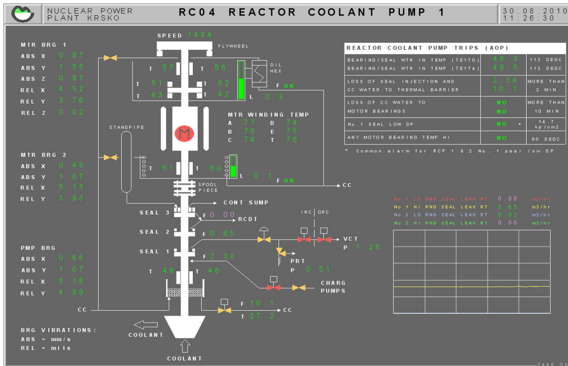
Slika 4.4 Kontinuirani monitoring reaktorske pumpe NEK-a
