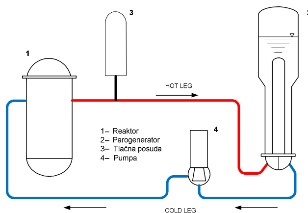
Slika 2.3 Komponente primarnog kruga
