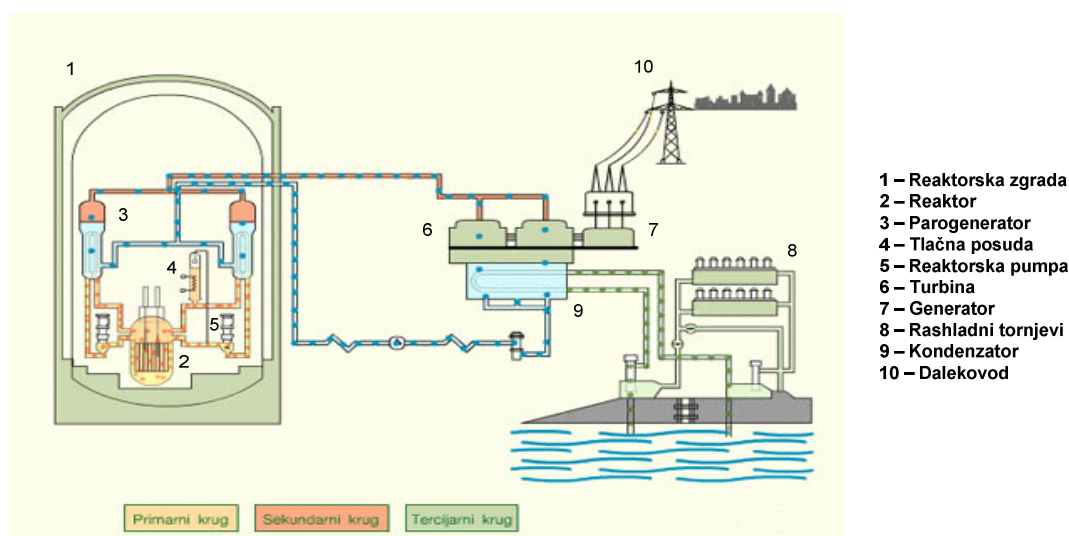
Slika 2.2 Shema NE s tlakovodnim reaktorom
