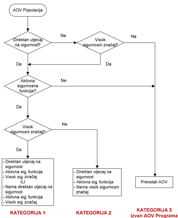
Slika 6.7 Princip kategorizacije AOV-a
