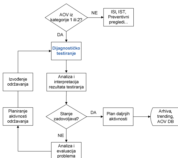
Slika 7.6 Pojednostavnjeni proces dijagnostike AOV-a
