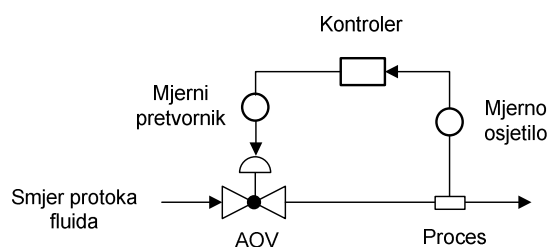
Slika 6.5 Regulacijski krug kontrolnog ventila
