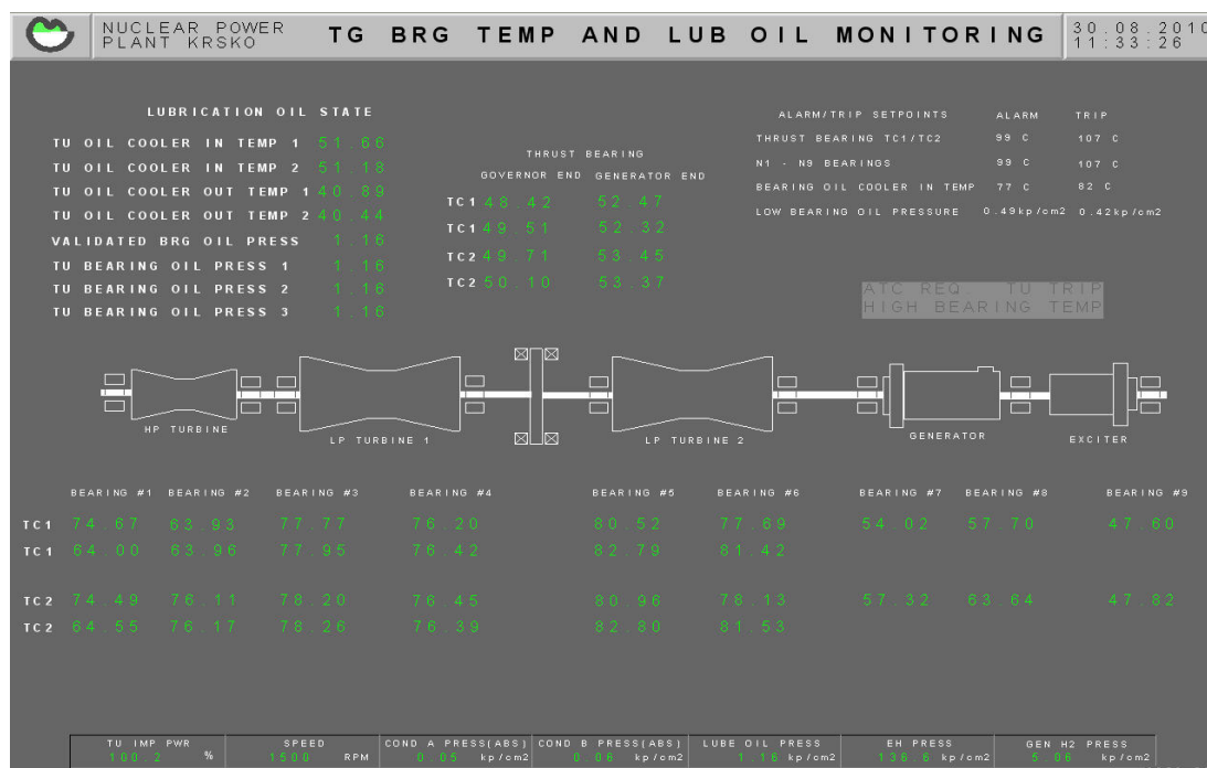
Slika 4.3 Kontinuirani monitoring turbine NEK-a
