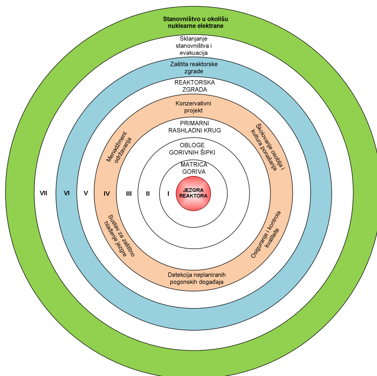
Slika 2.4 Zaštita okoliša po dubini
