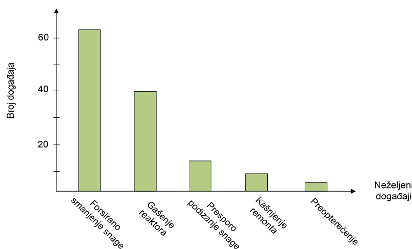
Slika 7.2 Utjecaj kvarova AOV-a na devijacije snage
