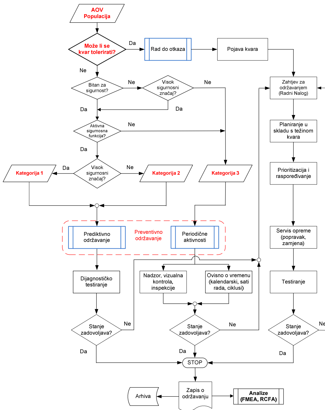
Slika 7.8 Predloženi koncept održavanja AOV-a
