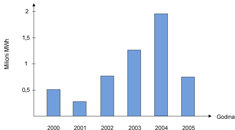
Slika 7.3 Gubici snage NE uzrokovani slabim performansama AOV-a
