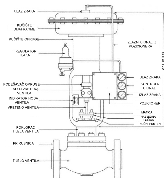
Slika 6.1 AOZ s pomoćnom opremom
