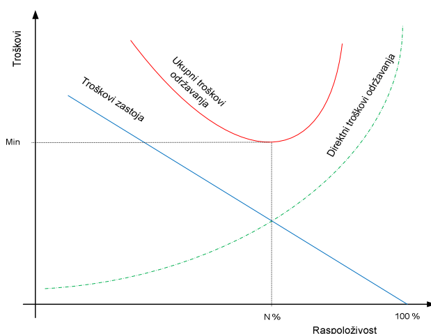
Slika 3.6 Odnos troškova održavanja i raspoloživosti TS-a
