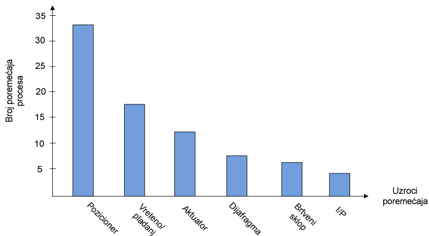
Slika 7.4 Frekvencija pojave kvara po komponentama AOV-a
