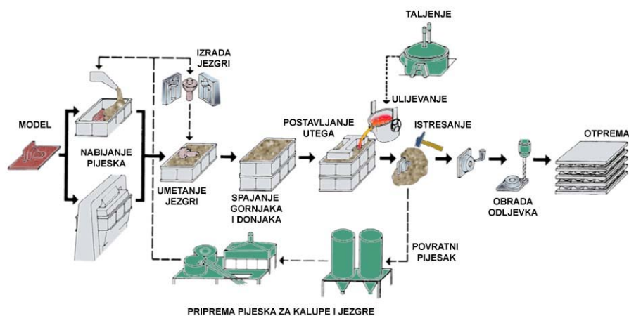
PROIZVODNI PROCES U LJEVAONICI
