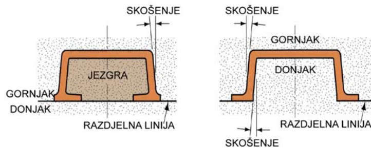
a) Izvorna konstrukcija
