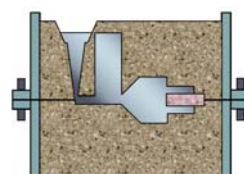
Zatvoreni kalup
