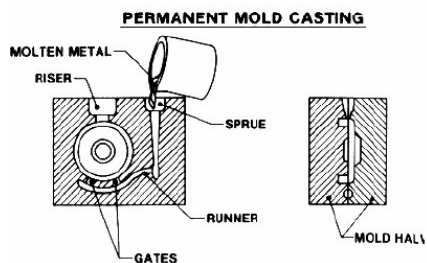
Gravitacijsko lijevanje u kokile
