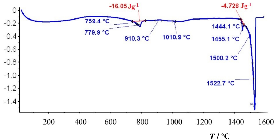
Slika 88. Termogram za uzorak alatnog čelika oznake HTCS-130 (zagrijavanje)
