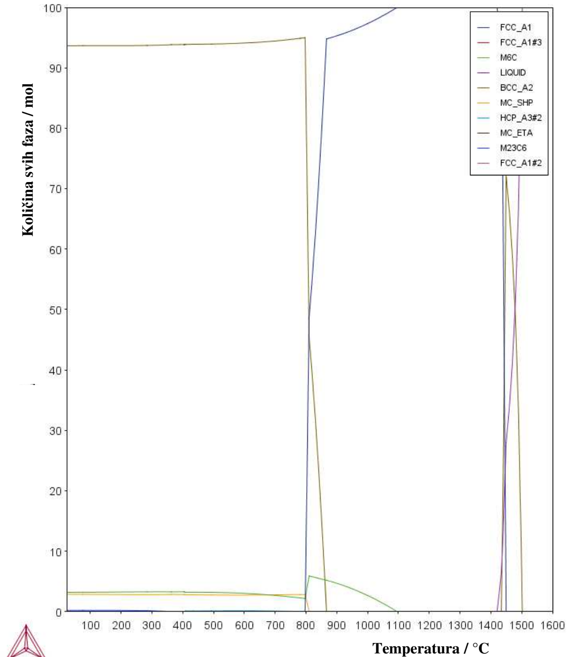
Slika 82. Fazni ravnotežni dijagram stanja (prikaz temperaturne stabilnosti faza pri ravnotežnim uvjetima za uzorak) HTCS-130
