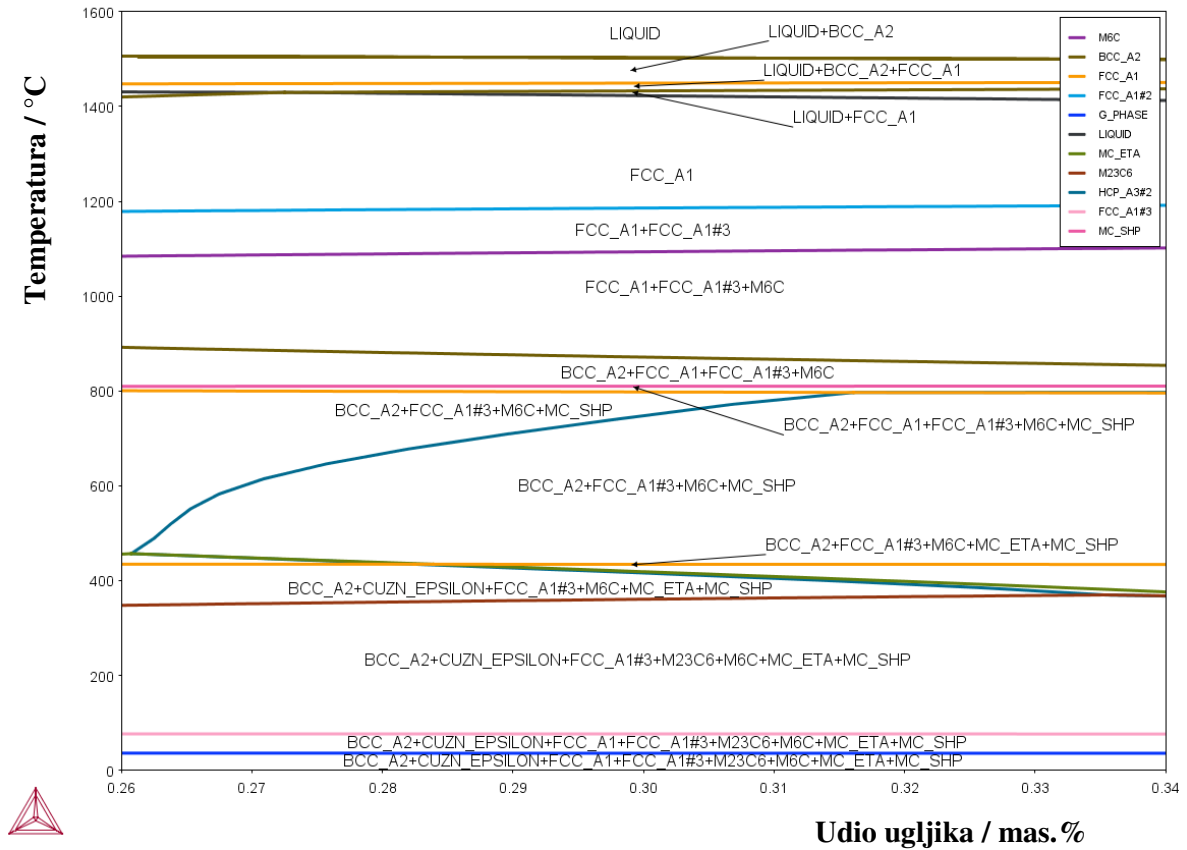
Slika 81. Izopletni ravnotežni fazni dijagram stanja alatnog čelika za topli rad oznake HTCS-
