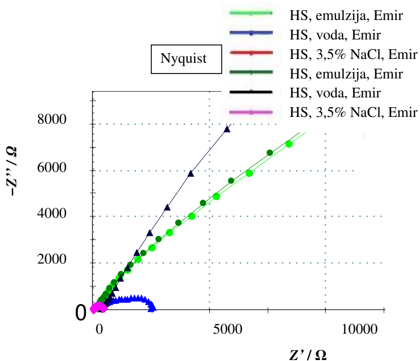
Slika 96. Komparativni prikaz Nyquistovih EIS spektara dobivenih za uzorke DS i HS ispitane u medijima Lenox Band-Ade emulzija, voda i 3,5 % NaCl
