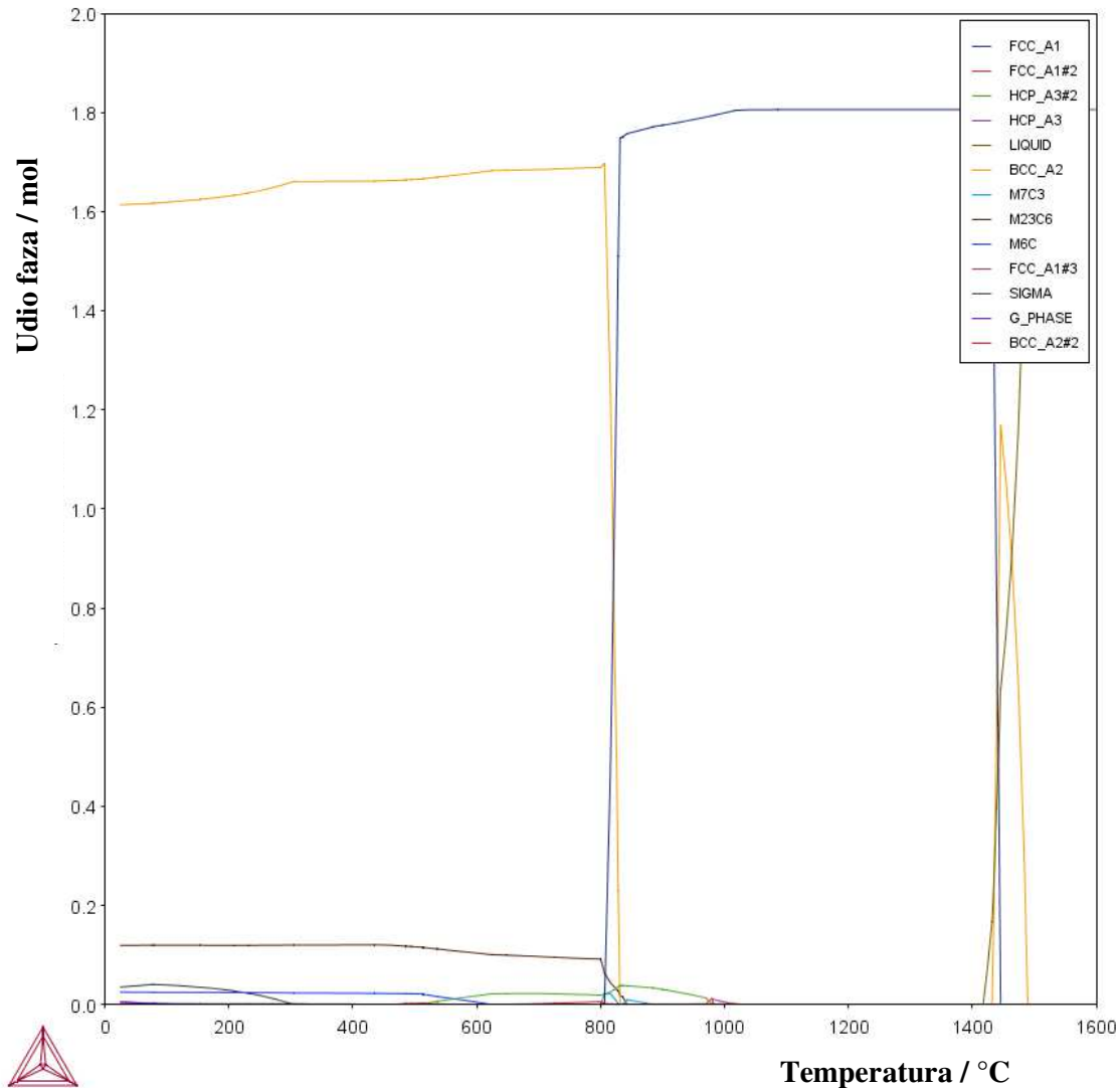
Slika 80. Fazni ravnotežni dijagram stanja (prikaz temperaturne stabilnosti faza pri ravnotežnim uvjetima) za uzorak Dievar
