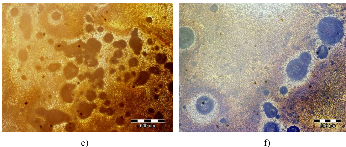
Slika 117. Metalografske snimke uzorka HS nakon elektrokemijskih ispitivanja u mediju emulzije Lenox Band-Ade: a) povećanje 50x i b) povećanje 100x, vodi: c) povećanje 50x i d) povećanje 100x, 3,5 % NaCl: e) povećanje 50x i f) povećanje 100x
