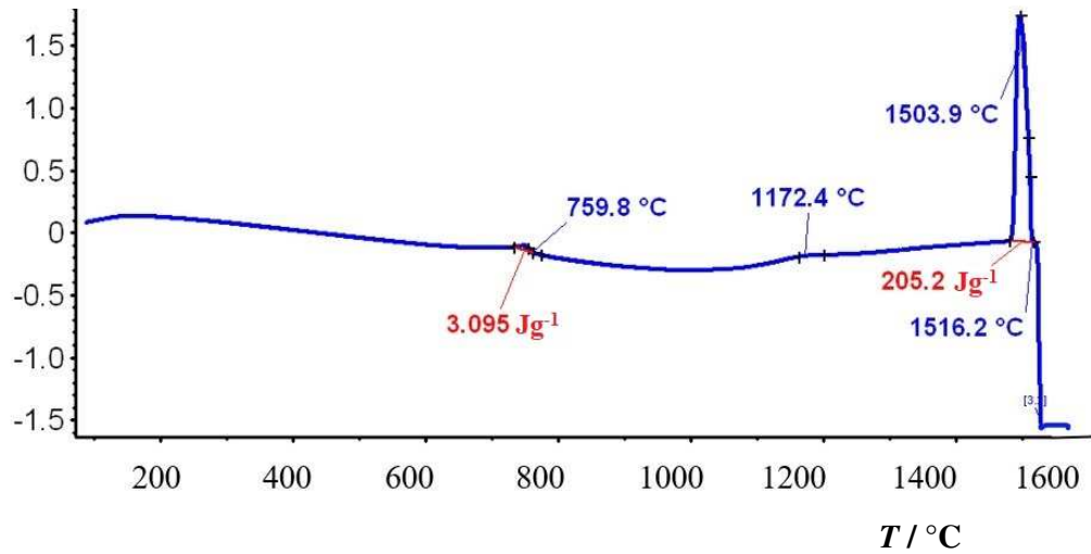
Slika 87. Termogram za uzorak alatnog čelika oznake Dievar (hlađenje)
