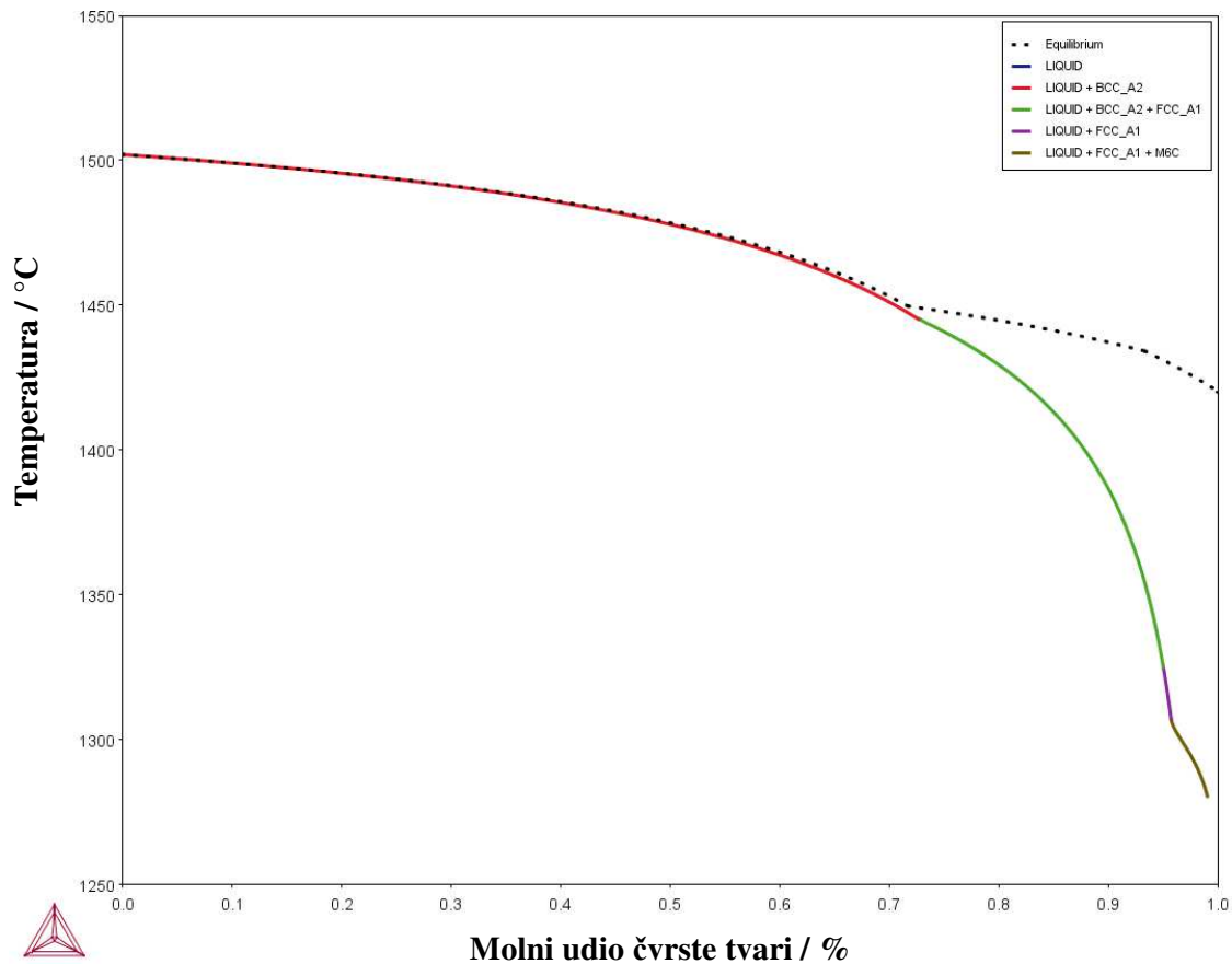
Slika 84. Scheil projekcija neravnotežnog skrućivanja za ispitivani alatni čelik HTCS-130
