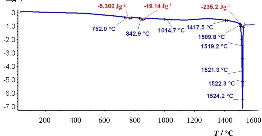
Slika 86. Termogram za uzorak alatnog čelika oznake Dievar (zagrijavanje)
