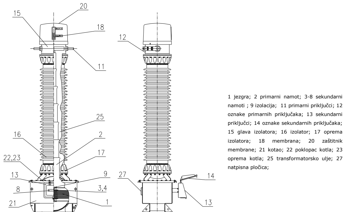
Slika 2 - 5: Uljni strujni transformator tipa APU-245
