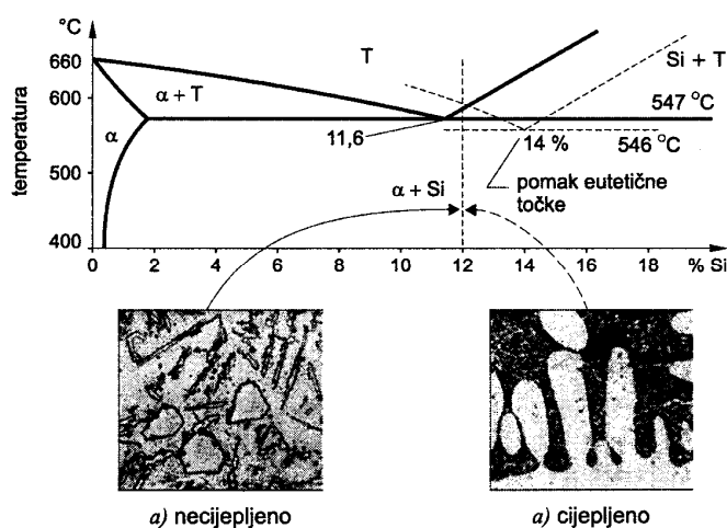
Slika 4 - 6: Dijagram stanja za Al-Si leguru [26]
