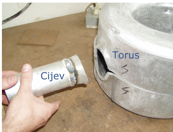
Slika 6 - 6: Uzorak 1 – odvojen od torusa
