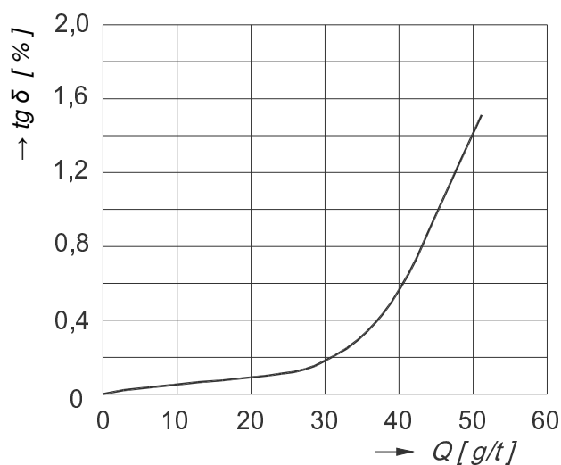
Slika 2 - 9: Faktor dielektričnih gubitaka [10]
