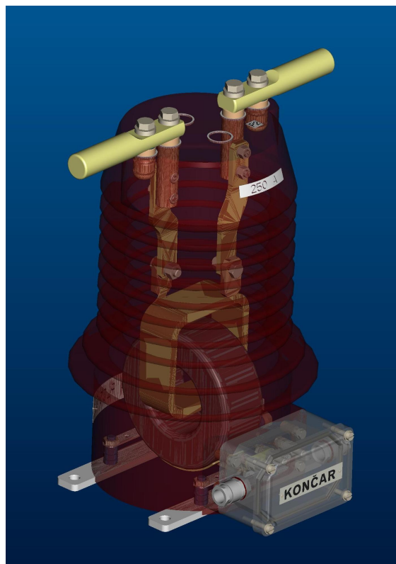
Slika 2 - 4: Epoksidni strujni transformator tipa APE 24
