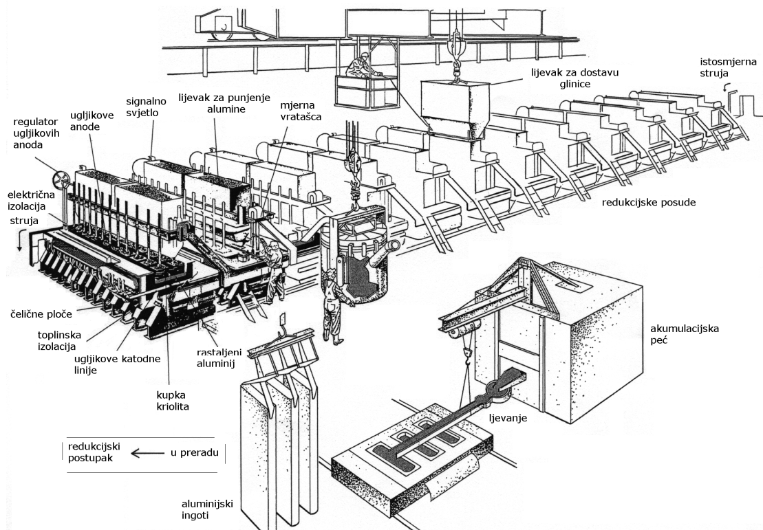
Slika 4 - 5: Postupak proizvodnje aluminija u talionici [33]
