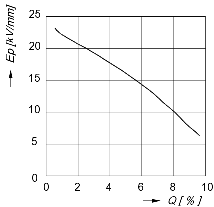
Slika 2 - 10: Dijagram 1-minutne efektivne vrijednosti dielektrične čvrstoće [10]
