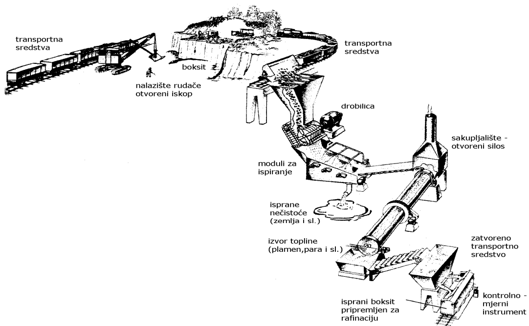
Slika 4 - 3: Postupak pripreme boksita za daljnju preradu [31]
