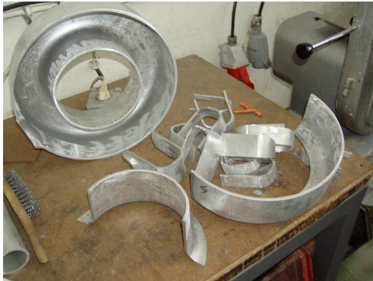
Slika 6 - 9: Izrezani dijelovi torusa – uzorak 2
