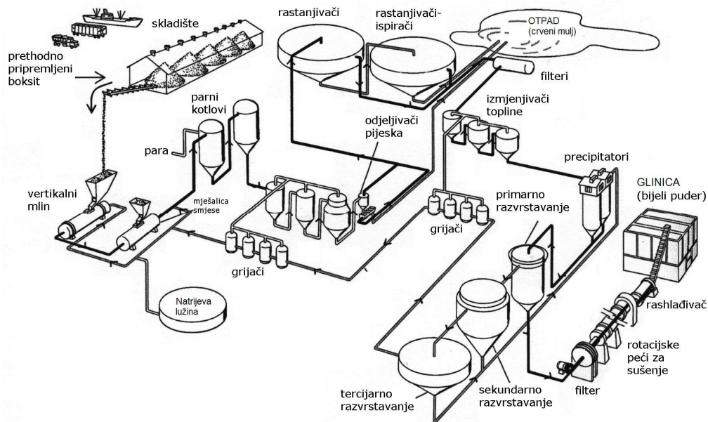
Slika 4 - 4: Postupak dobivanja glinice iz boksita [31]
