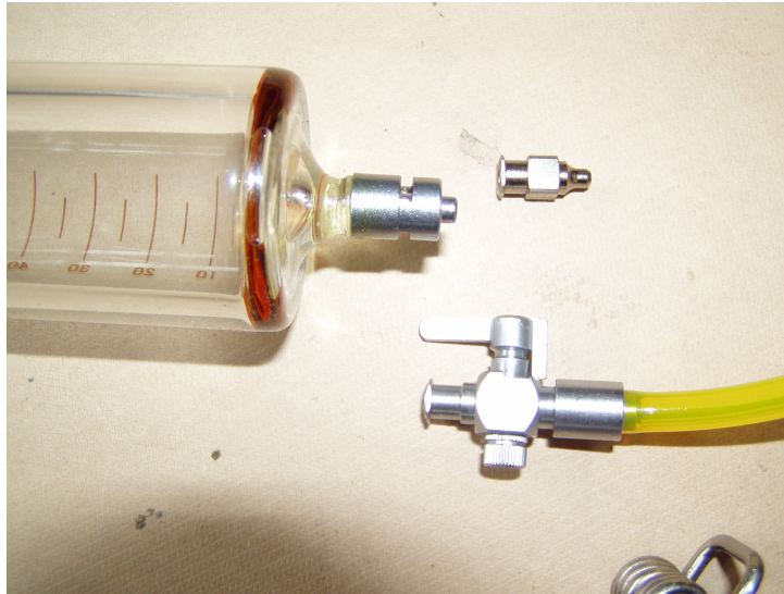
Slika 3 - 3: Sistem „luer lock“ na otvoru šprice sa pripadajućim čepom i ventilićem
