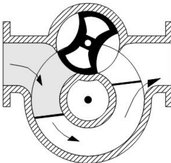
Slika 2.10: Plinomjer s rotirajućim komorama
