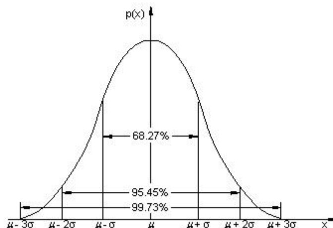
Slika 4.4: Odnos između funkcije gustoće vjerojatnosti i njenih statističkih parametara, \mu i \sigma
