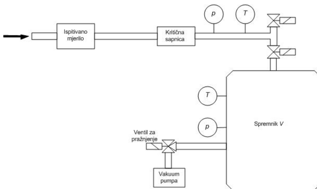
Slika 2.5: pVT-t sustav
