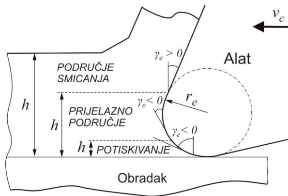
Slika 2.16 Utjecaj zaobljenja rezne oštrice alata i debljine deformirane čestice na efektivni kut prednje površine alata
