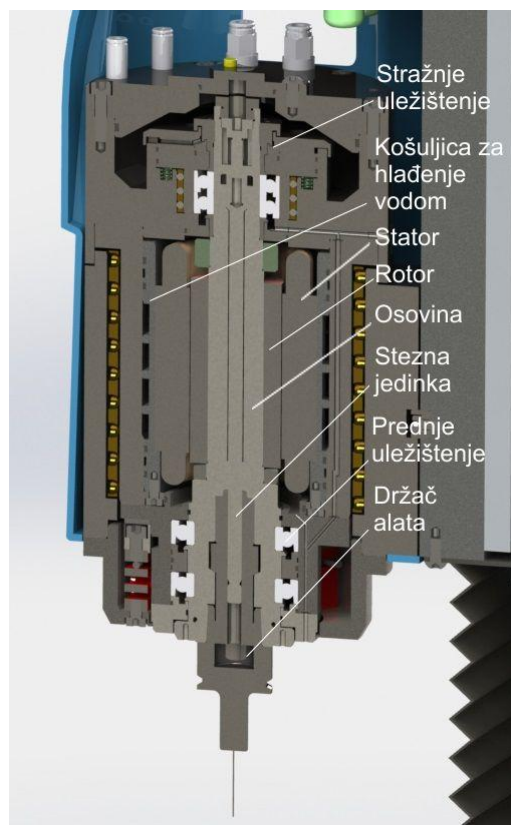
Slika 4.3 Motorvreteno HSTEC-HSM080AA-V01-LK719-55
