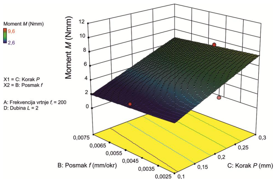
Slika 5.17 3D prikaz matematičkog modela ovisnosti momenta M mikrobušenja o posmaku f i dubini koraka P (dubina provrta L = 2 mm, n = 12\,000\text{ min}^{-1} )
