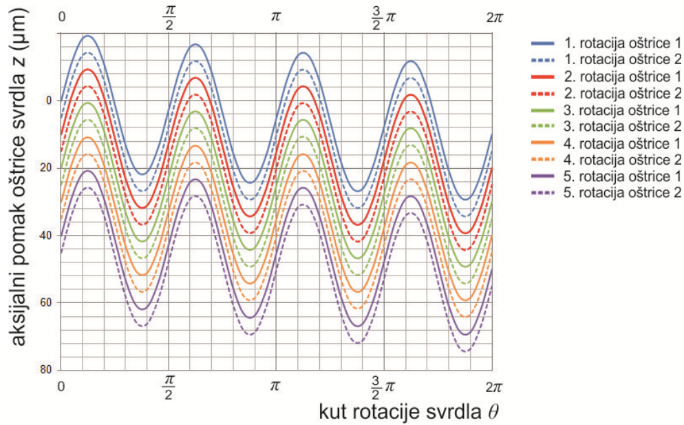
Slika 3.7 Trajektorije dviju oštrica kod bušenja potpomognutoga vibracijama ( f = 10 \mu\text{m/okr} , r_f = 4 , A = 20 \mu\text{m} )
