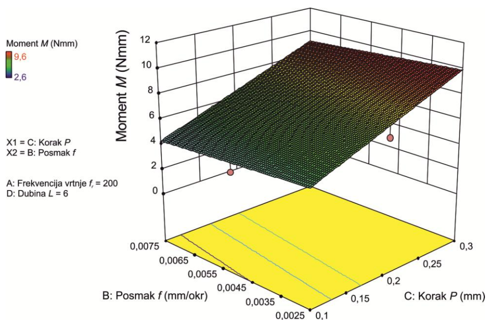
Slika 5.18 3D prikaz matematičkog modela ovisnosti momenta M mikrobušenja o posmaku f i dubini koraka P (dubina provrta L = 6 mm, n = 12\,000\text{ min}^{-1} )
