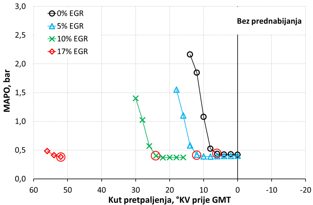
Slika 4.9. MAPO u ovisnosti o kutu prepaljenja za radne točke bez prednabijanja
