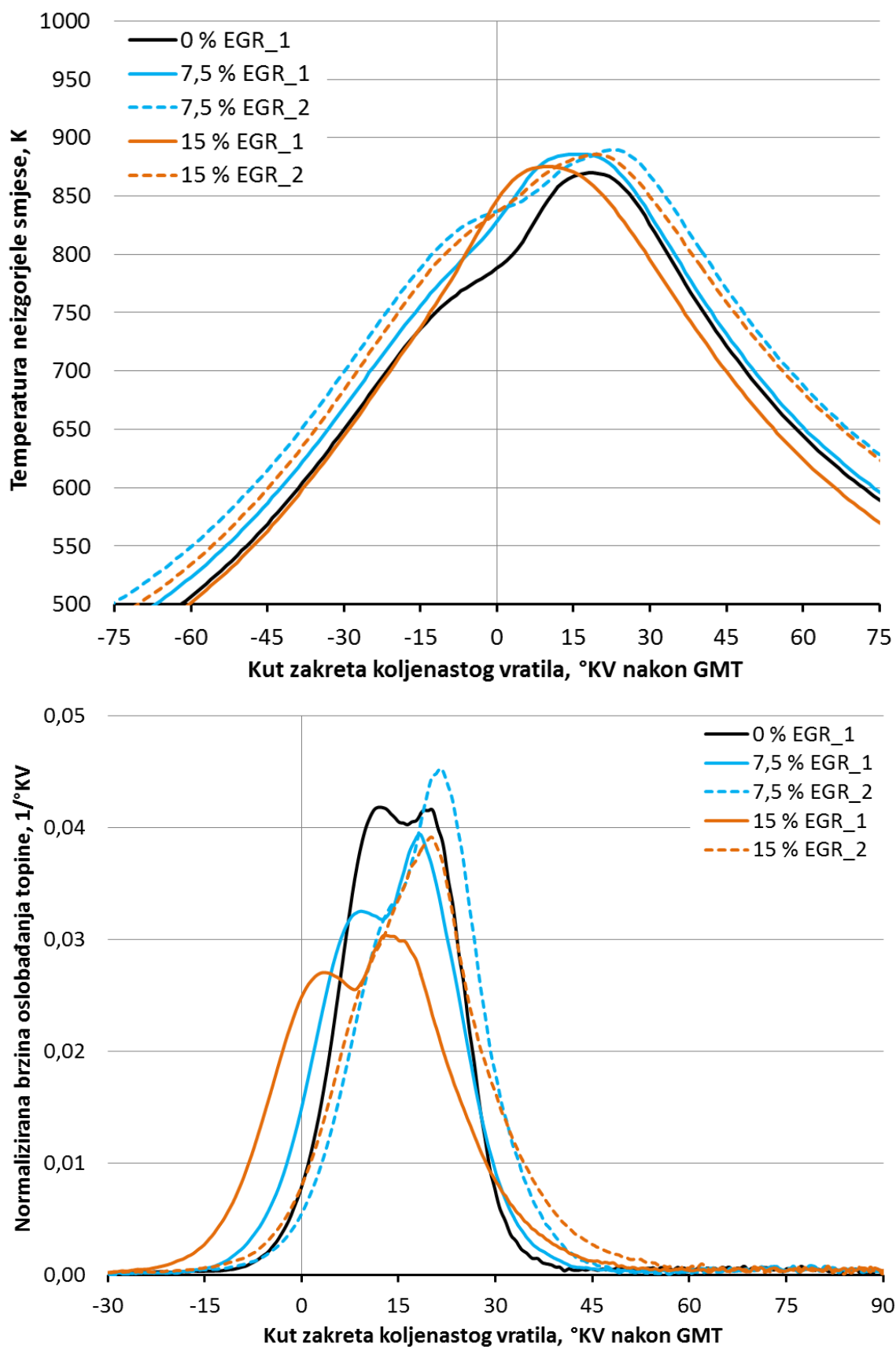
Slika 5.27. Profili temperature neizgorjele smjese i normalizirane brzine oslobađanja topline
