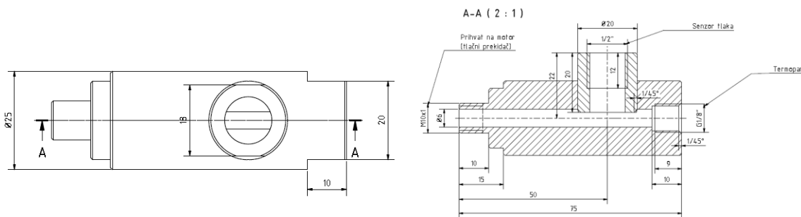
Slika 2.14. Prihvati senzora tlaka i temperature ulja
