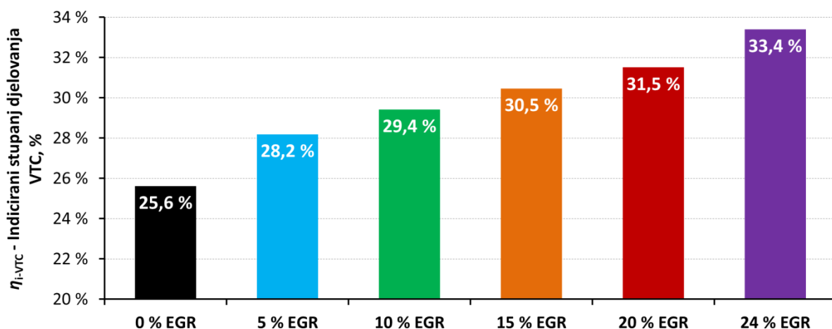
Slika 5.39. Indicirani stupanj djelovanja visokotlačnog dijela radnog ciklusa motora za radne točke s prednabijanjem u ovisnosti o udjelu EGR-a
