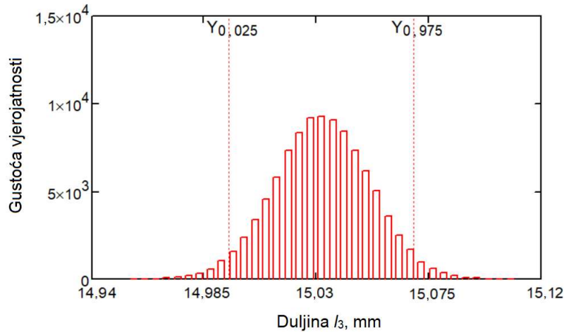
Slika 5-11. Funkcija gustoće vjerojatnosti g(l_3) vanjskog promjera polimernog cilindra složene geometrije.
