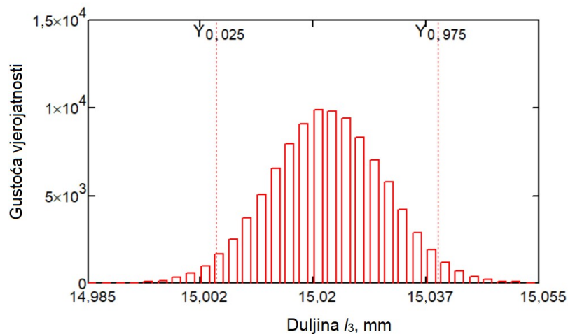
Slika 5-6. Funkcija gustoće vjerojatnosti g(l_3) vanjskog promjera aluminijskog cilindra složene geometrije.
