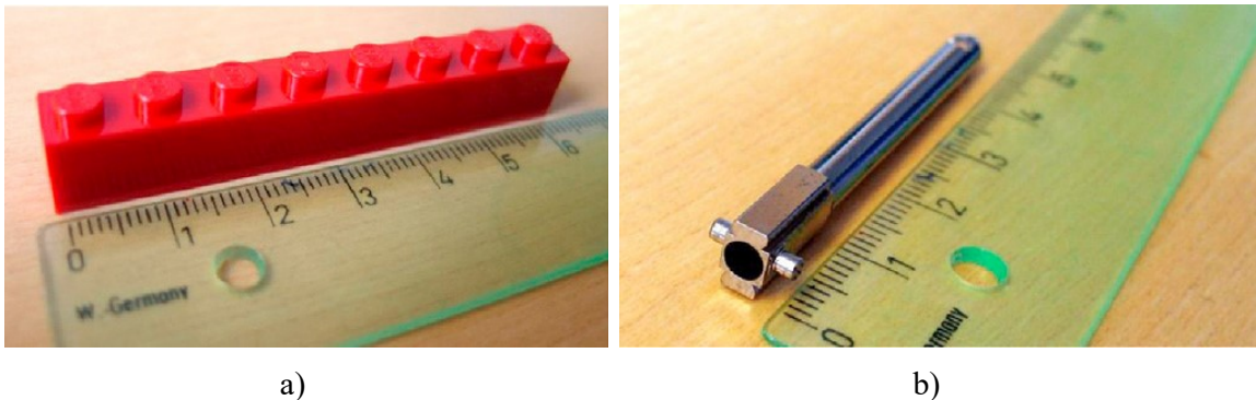
Slika 3-14. Referentni predmeti korišteni u interkomparaciji CIA-CT: a) LEGO kocka, b) komponenta inzulinske olovke [82].
