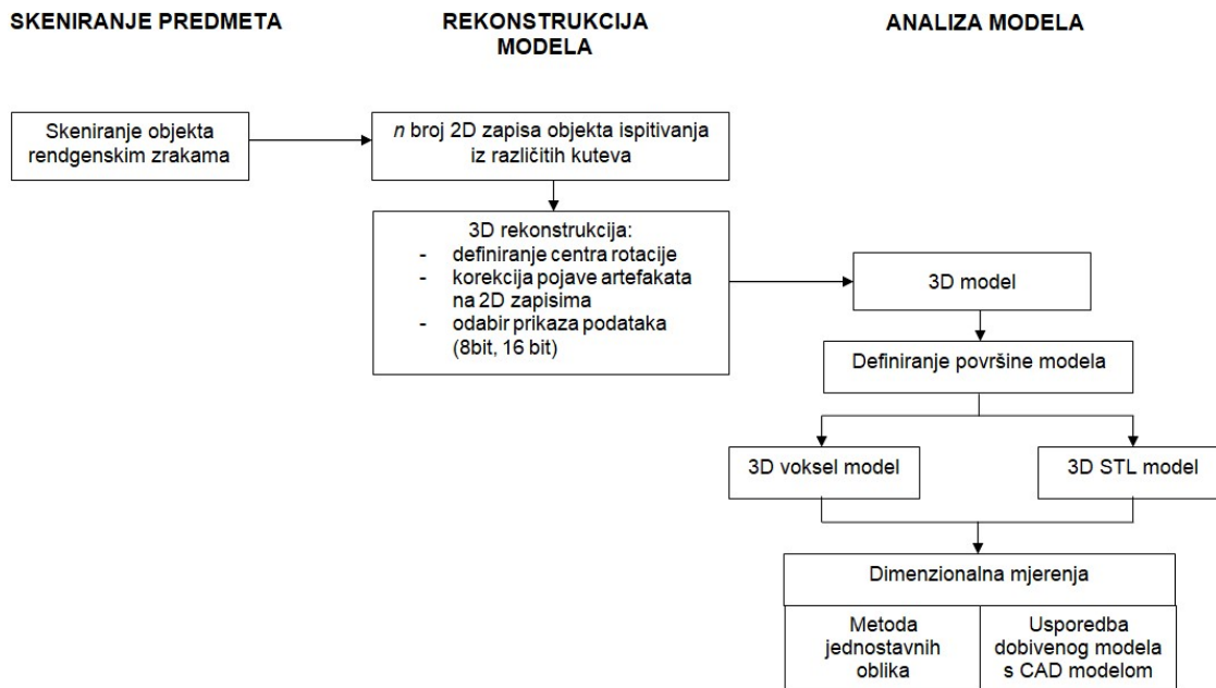
Slika 2-2. Proces provedbe dimenzionalnog mjerenja računalnom tomografijom.
