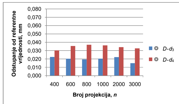
Slika 4-12. Odstupanje od koaksijalnosti s povećanjem broja projekcija.
