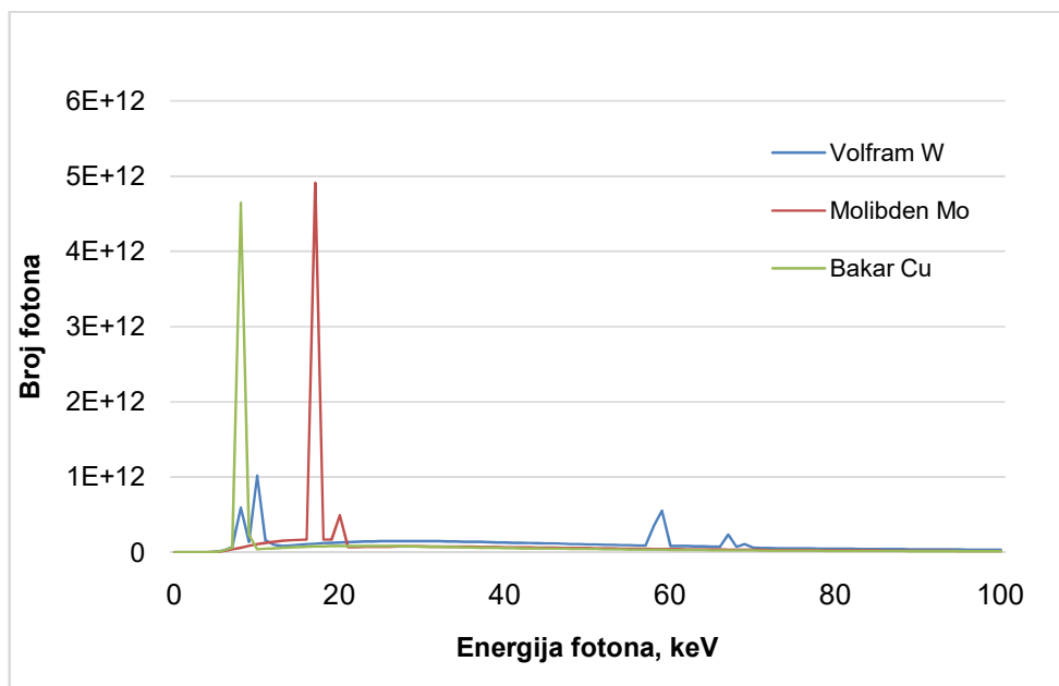
Slika 2-10. Spektar rendgenskog zračenja za različite materijale anode.
