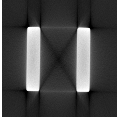
Slika 2-19. Artefakti otvrdnjavanja zračenja u obliku crta.
