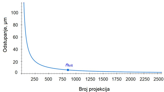
Slika 4-5. Odstupanje u ovisnosti o broju projekcija prema teorijski pretpostavljenoj funkciji.
