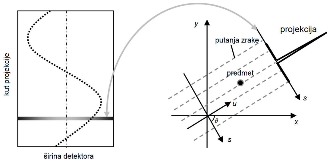
Slika 2-15. Formiranje sinograma [10].
