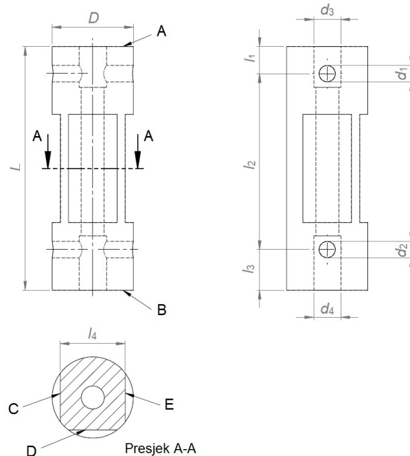
Slika 4-4. Crtež cilindra složene geometrije.
