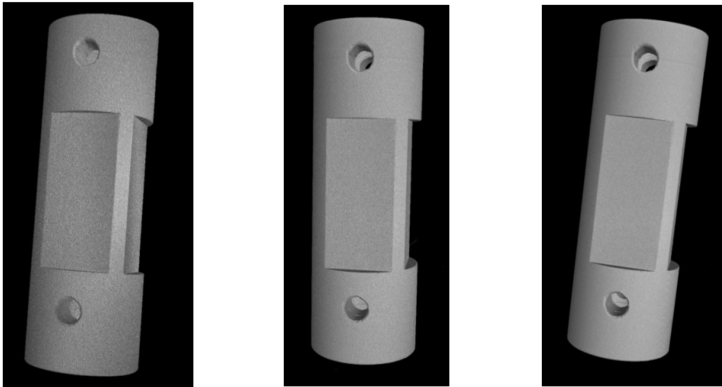
a) b) c) Slika 4-7. Rekonstruirani modeli za različiti broj 2D projekcija:
