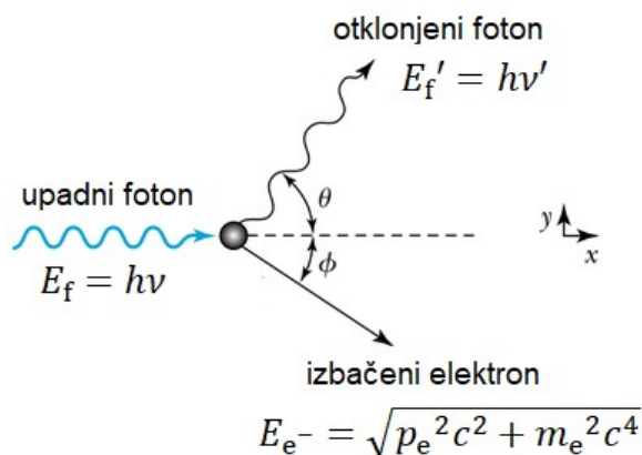
Slika 2-21. Nekoherentno zračenje [39].
