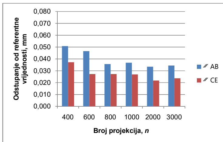
Slika 4-10. Odstupanje paralelnosti s povećanjem broja projekcija.
