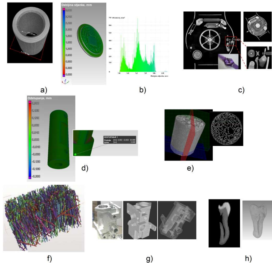
Slika 2-1. Primjena industrijske računalne tomografije
