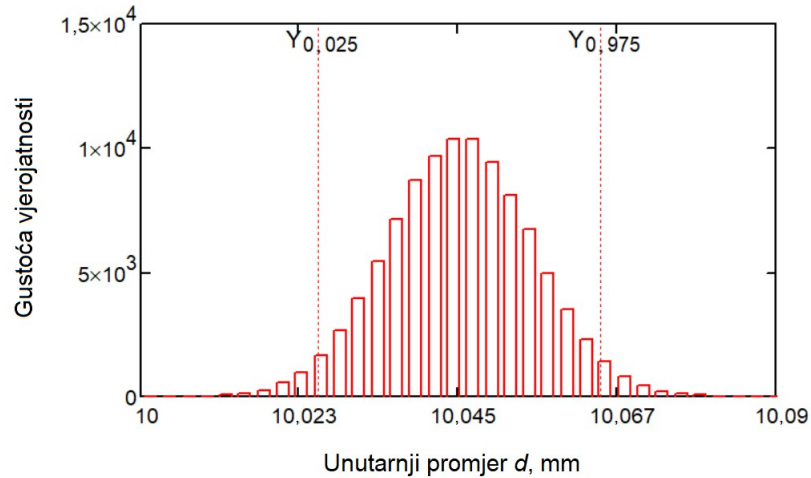
Slika 5-9. Funkcija gustoće vjerojatnosti g(d_3) unutarnjeg promjera polimernog cilindra složene geometrije.
