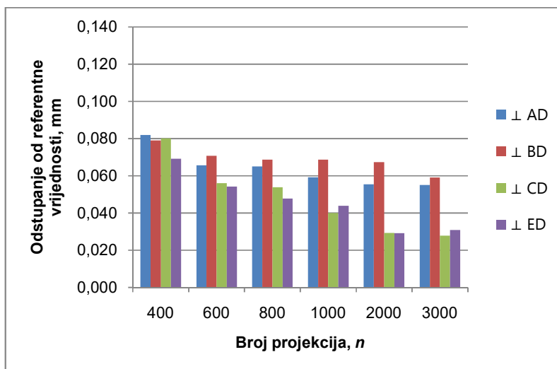
Slika 4-9. Odstupanje od okomitosti s povećanjem broja projekcija.
