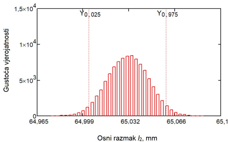
Slika 5-12. Funkcija gustoće vjerojatnosti g(l_2) vanjskog promjera polimernog cilindra složene geometrije.
