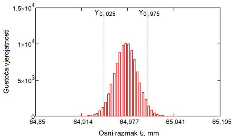
Slika 5-7. Funkcija gustoće vjerojatnosti g(l_2) vanjskog promjera aluminijskog cilindra složene geometrije.
