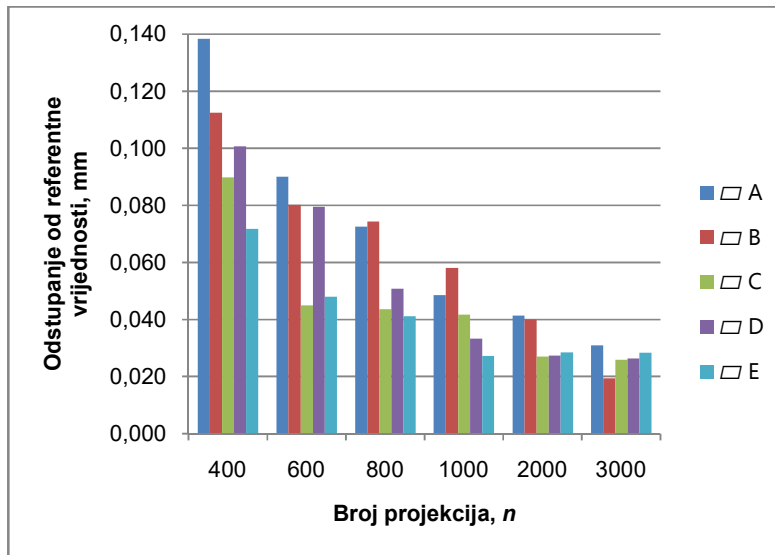
Slika 4-8. Odstupanje od ravnosti s povećanjem broja projekcija.
