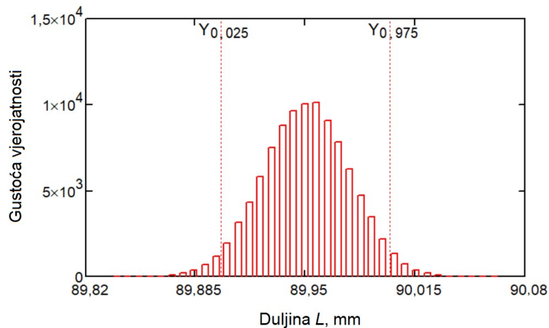
Slika 5-10. Funkcija gustoće vjerojatnosti g(L) polimernog cilindra složene geometrije.
