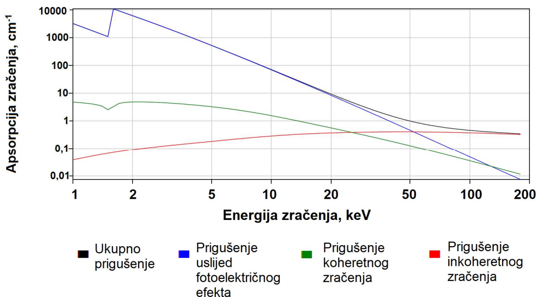
Slika 2-13. Koeficijenti prigušenja monokromatskog rendgenskog zračenja za aluminij.
