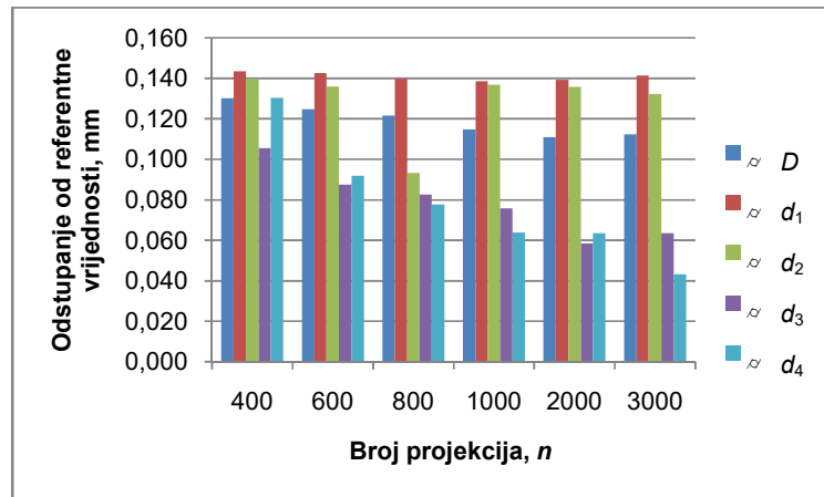
Slika 4-11. Odstupanje od cilindričnosti s povećanjem broja projekcija.
