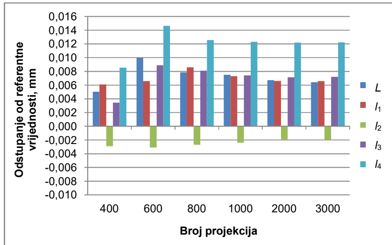
Slika 4-14. Odstupanje udaljenosti L , l_1 , l_2 , l_3 i l_4 s povećanjem broja projekcija.
