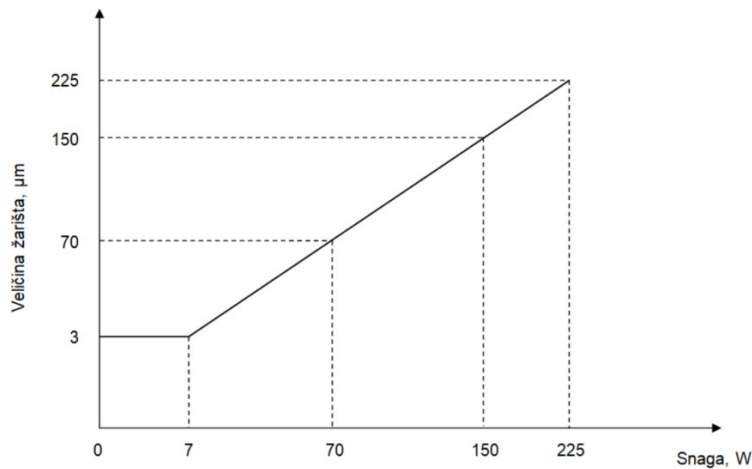
Slika 4-30. Relacija veličine žarišta i snage izvora zračenja.
