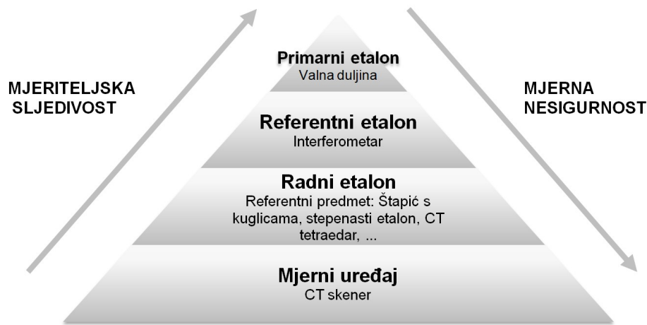
Slika 3-1. Lanac sljedivosti kod industrijske računalne tomografije.
