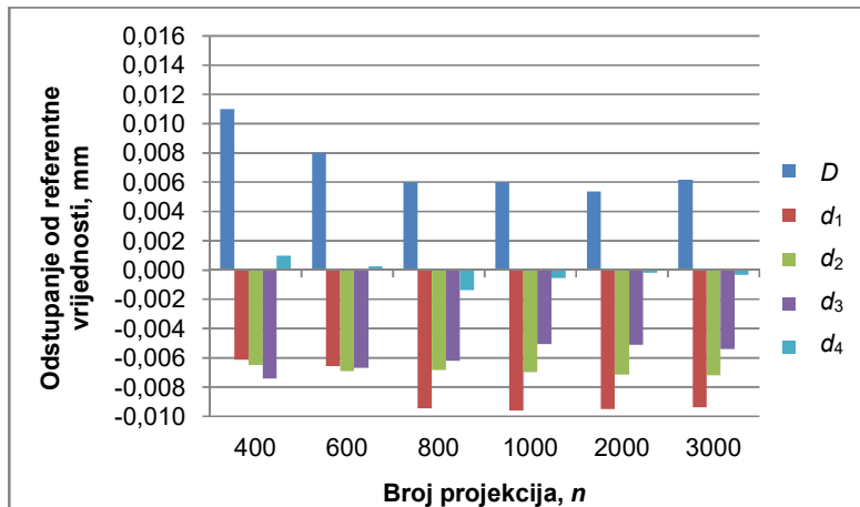
Slika 4-13. Odstupanje rezultata mjerenja vanjskog i unutarnjih promjera s povećanjem broja projekcija.
