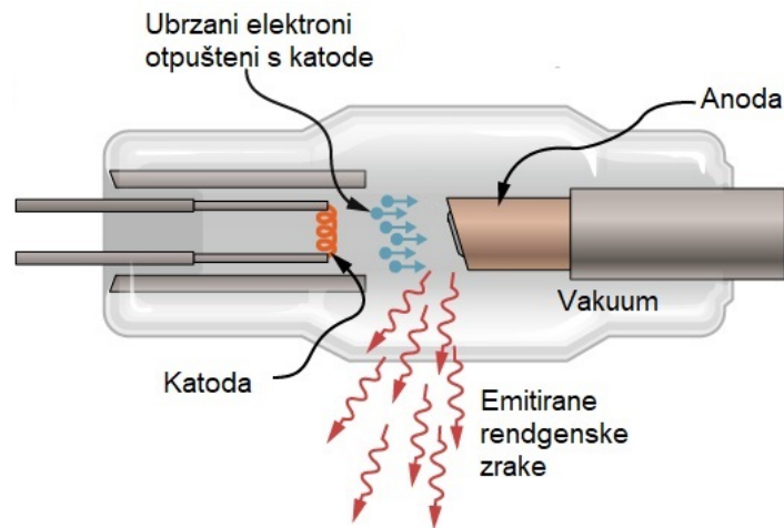
Slika 2-7. Rendgenska cijev [16].
