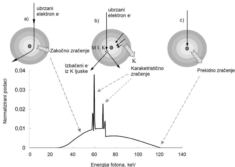
Slika 2-8. Nastajanje spektra rendgenskog zračenja[10].
