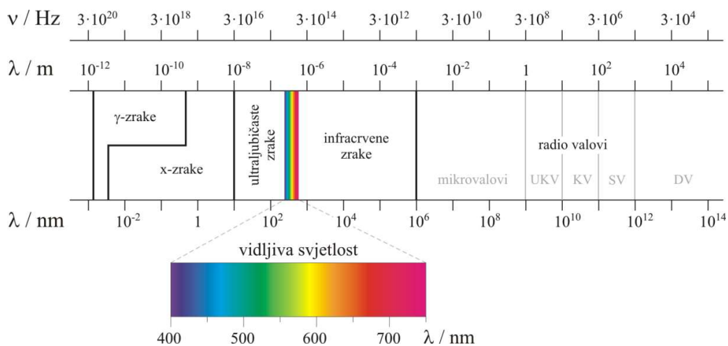
Slika 2-6. Spektar elektromagnetskog zračenja [15].
