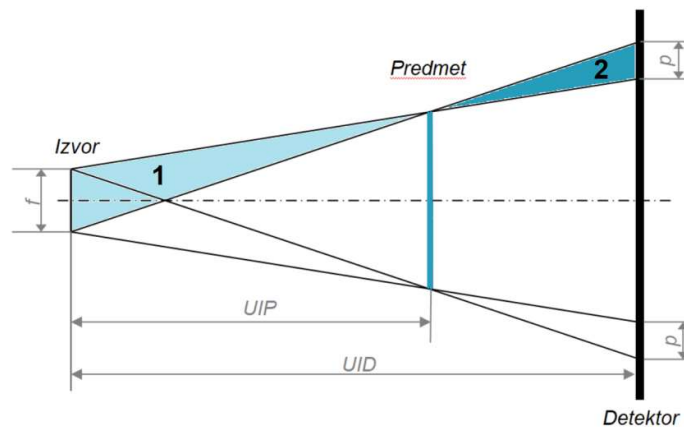
Slika 4-32. Efekt polusjene.
