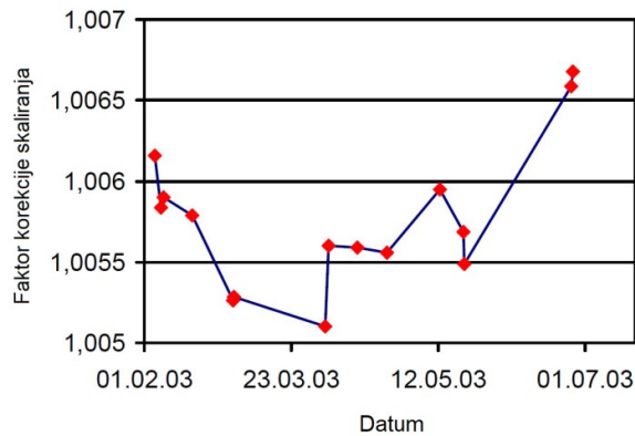
Slika 4-35. Promjena faktora korekcije skaliranja u razdoblju od 5 mjeseci [102].
