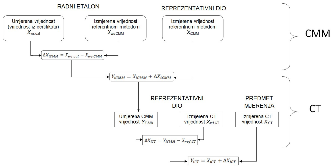
Slika 3-12. Postupak provedbe dimenzionalnih mjerenja sukladno ISO 15530-3 [77].
