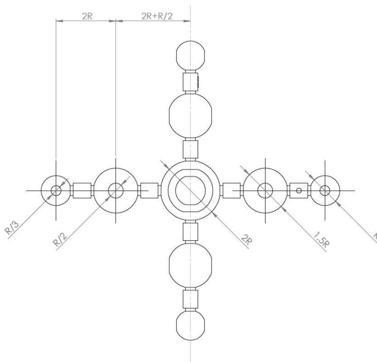
Slika 3-8. Crtež referentnog predmeta s definiranim dimenzijama.
