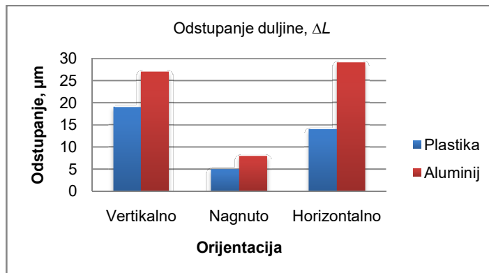
Slika 4-16. Odstupanja rezultata mjerenja duljine L kod različitih orijentacija polimernog i aluminijskog cilindra.
