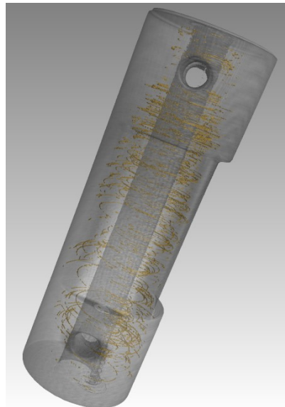
Analiza pora - cirkularni artefakti
