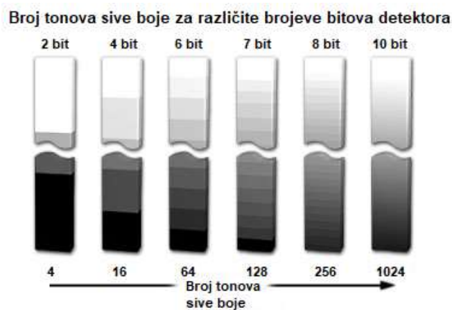
Slika 2-14. Broj različitih vrijednosti sivih tonova za različite brojeve bitova detektora. [25].
