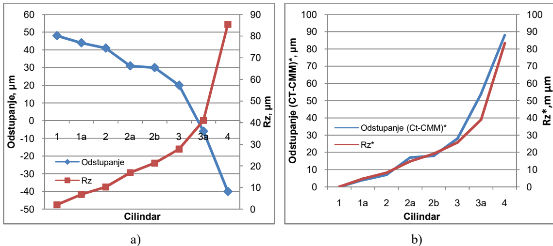
Slika 4-28. Rezultati dimenzionalnih mjerenja promjera vanjskog cilindra 8 cilindara u odnosu na izmjerenu hrapavost Rz : a) prije korekcije rezultata, b) nakon korekcije rezultata.
