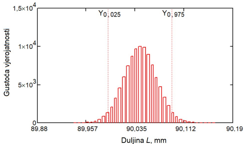
Slika 5-5. Funkcija gustoće vjerojatnosti g(L) aluminijskog cilindra složene geometrije.
