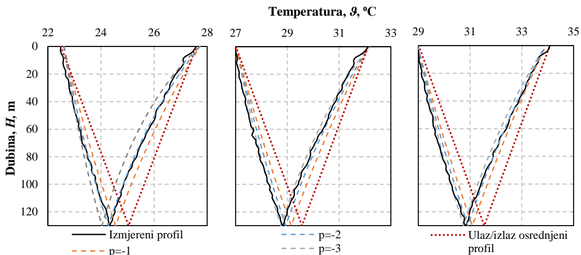
Slika 5-17 Profil temperature izmjerene kabelom s optičkim vlaknom (crna linija) te aproksimacije aritmetičkom sredinom te p-linearom metodom (lijevo 10. sat, sredina 50. sat, desno 100. sat)
