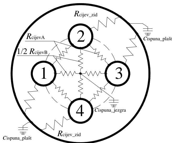
Slika 6-4 Presjek BIT-a s pripadnim toplinskim otporima i toplinskim kapacitetima ispunje
