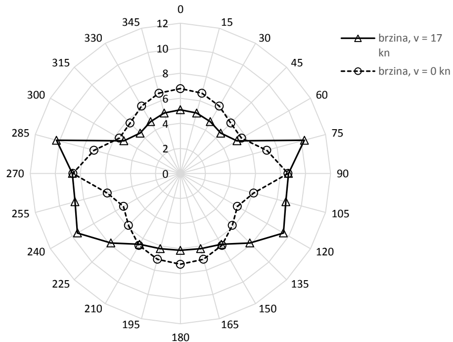
Slika 7-7 Polarni dijagram granične značajne valne visine H_s [m] obzirom na relativni kurs broda u odnosu na valove prema kriteriju udaranja pramca
