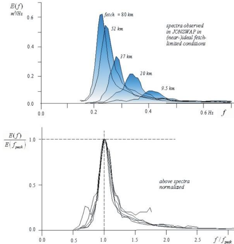
Slika 6-6 Razvoj JONSWAP spektra u kojem je modalna frekvencija izražena ovisno o brzini vjetra i duljini privjetrišta Izvor: Holthuijsen LH. Waves in oceanic and coastal waters. Cambridge university press; 2010 Feb 4.
