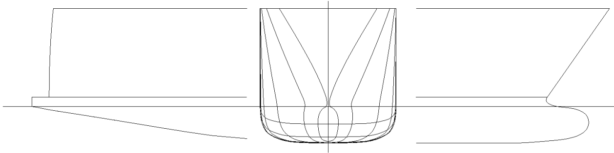
Slika 7-2 Linije broda za analizu pomorstvenosti
