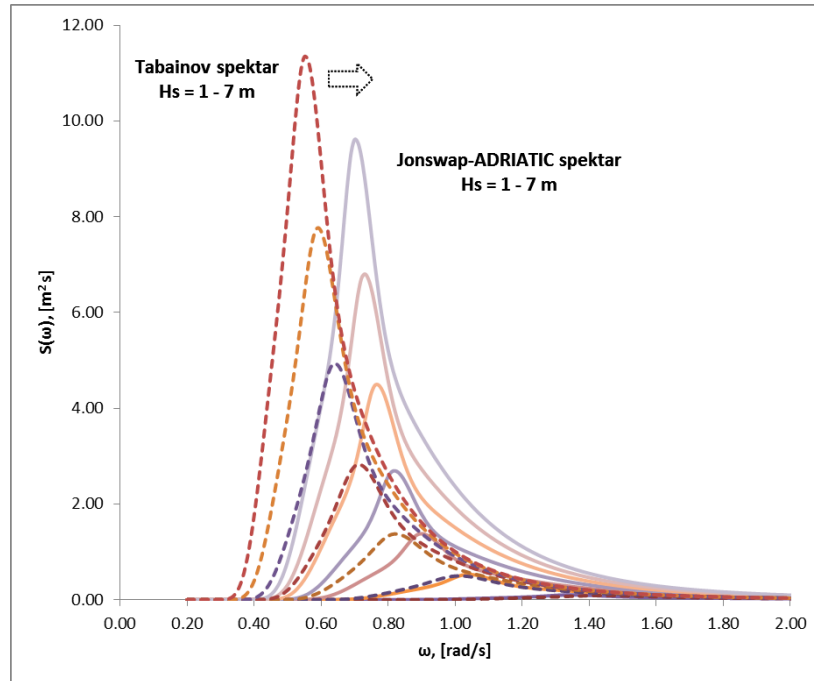
Slika 6-9 Transformacija Tabainovog spektra valova u JONSWAP-Adriatic spektr za unaprijedi opis valova Jadranskog mora na temelju rezultata numeričkih re-analiza i mjerenja satelitskom altimetrijom
