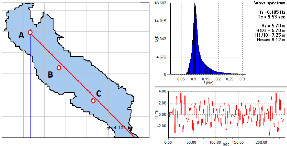
Slika 4-13 cgWindWaves (Runet 2016) domena i privjetrište za utvrditi H_s (lijevo), spektralni opis (gore desno) te primjer mogućeg valnog zapisa u vremenskoj domeni (dolje desno) za Lokaciju A, JI vjetar = 20 m/s
