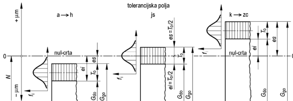
Slika 4.4. Položaj tolerancijskih polja kod vanjske izmjere (osovine) i učestalost pojave stvarnih izmjera
