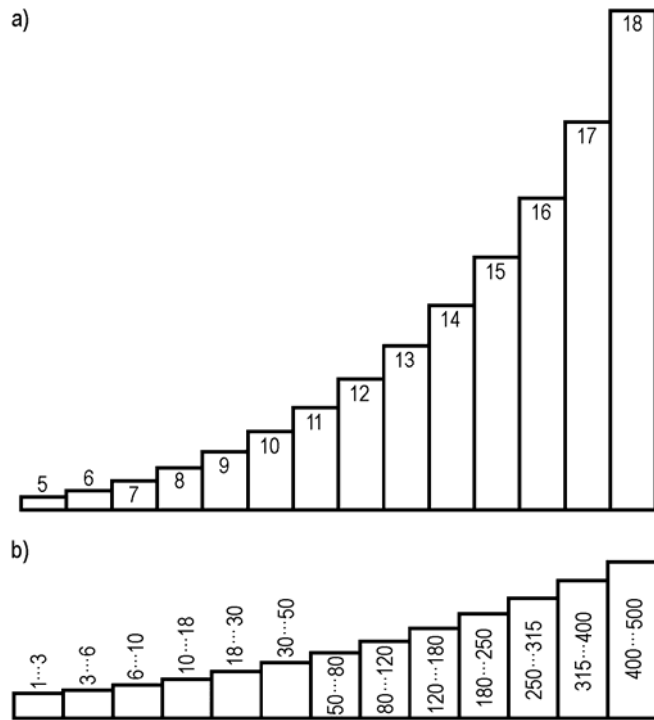
Slika 4.11. Promjena veličine tolerancijskog polja (a - ovisno o kvaliteti tolerancije i b - ovisno o području nazivne izmjere)
