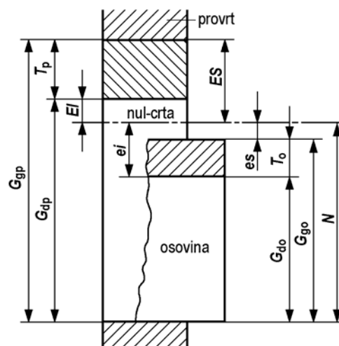
Slika 4.1. Definicija osnovnih pojmova tolerancija izmjera
